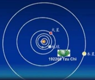
慈濟小行星軌道圖
